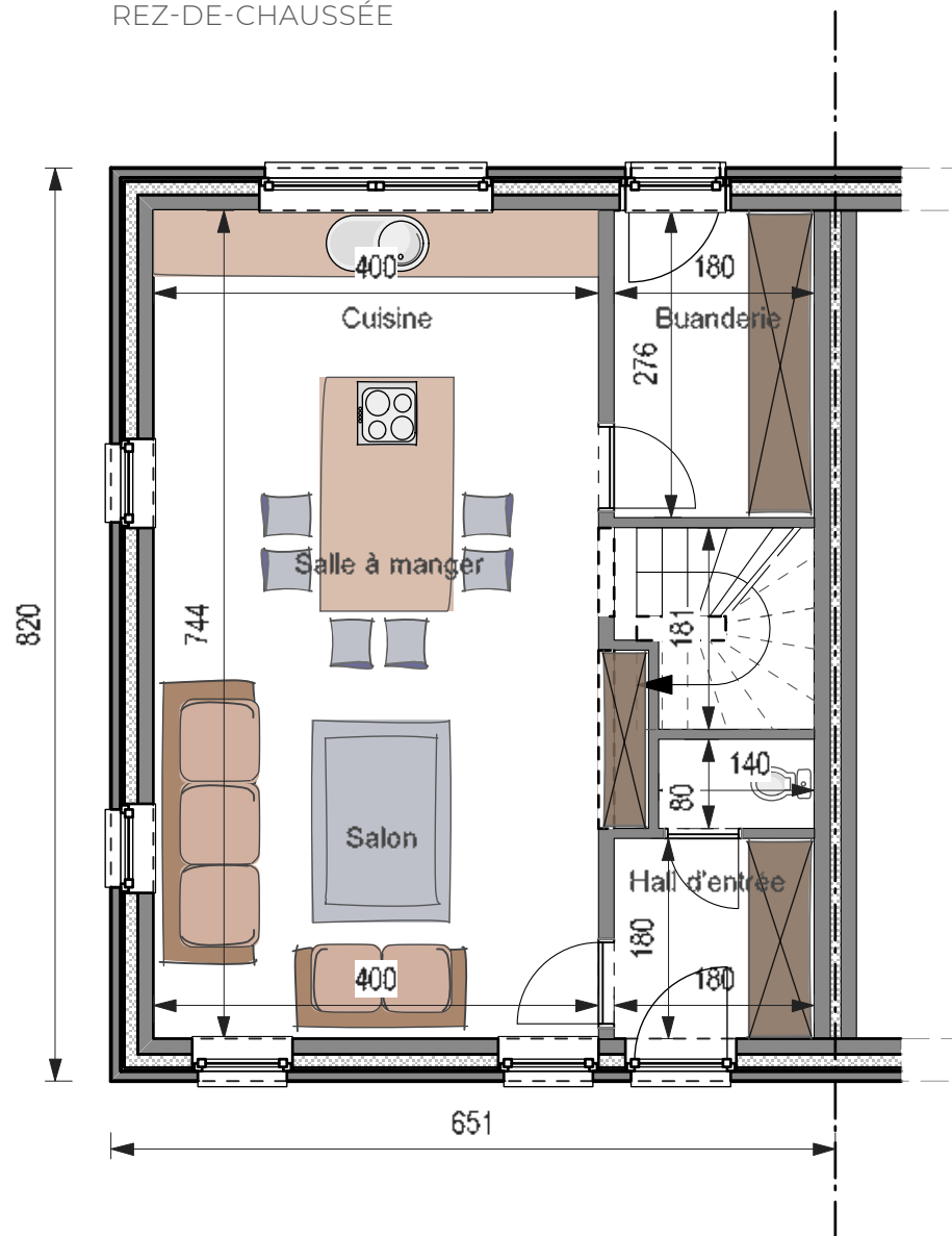
REZ-DE-CHAUSSÉE
