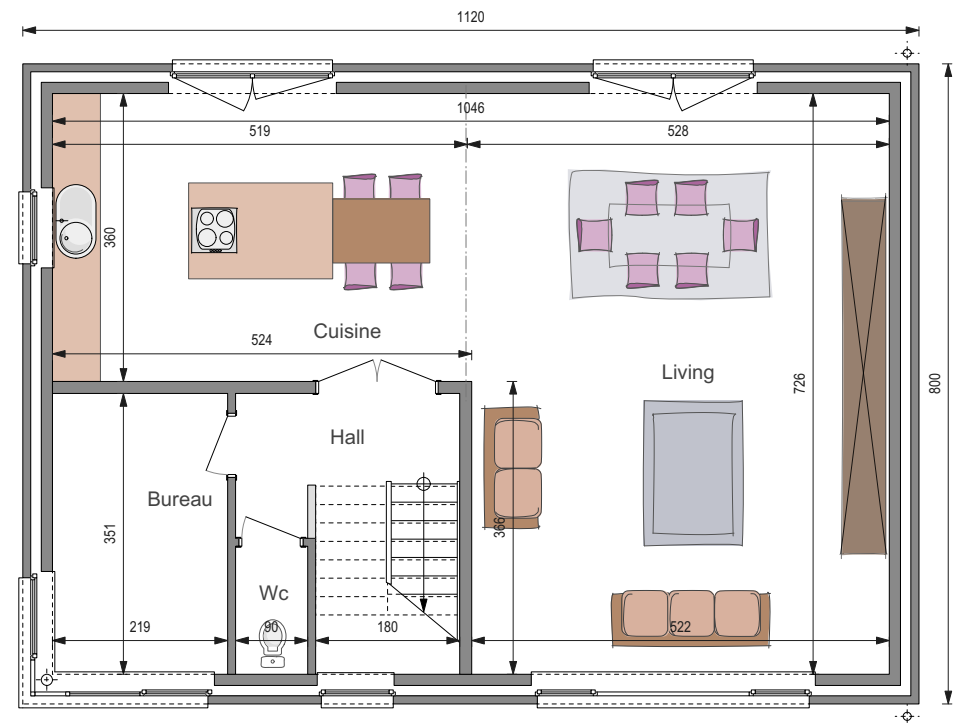
ÉTAGE 1
