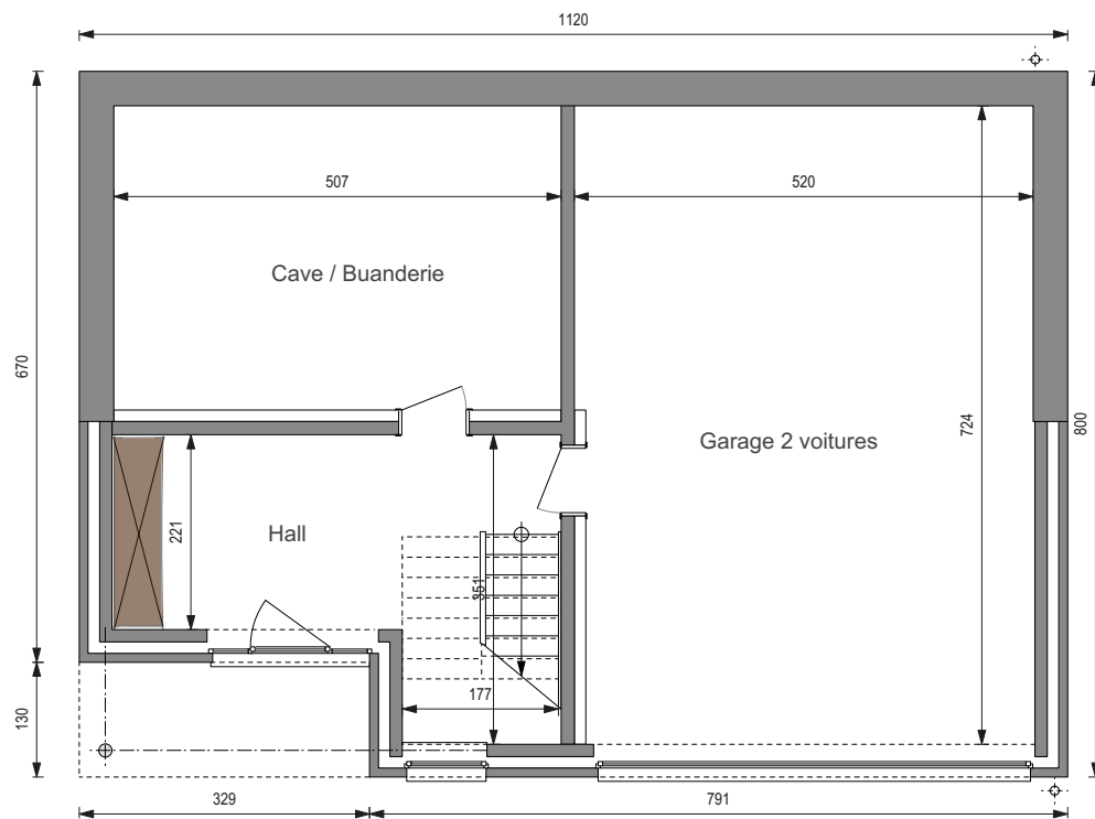
REZ-DE-CHAUSSÉE
