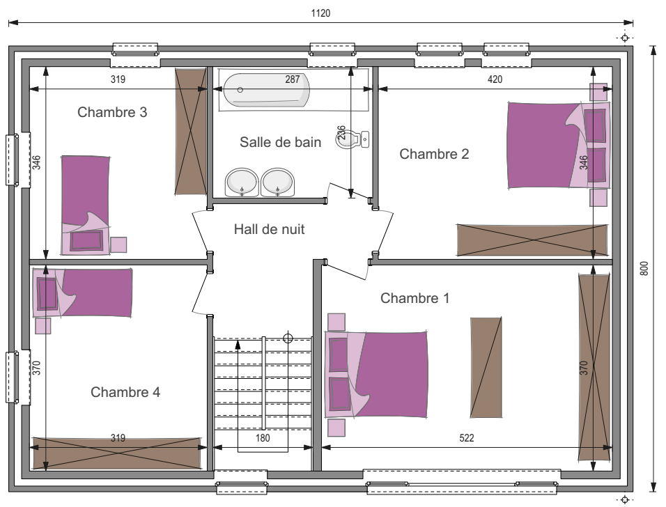
ÉTAGE 2
