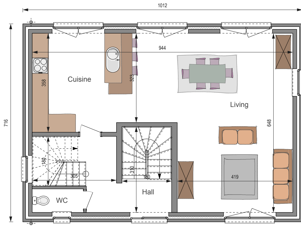
ÉTAGE 1
