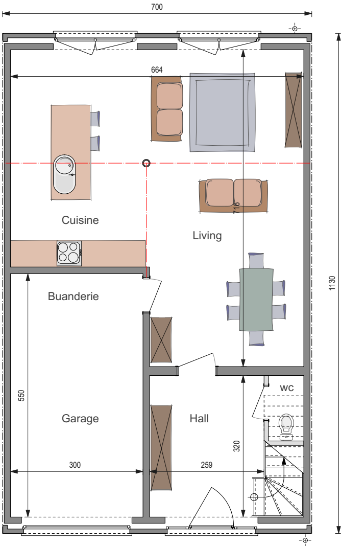
REZ-DE-CHAUSSÉE
