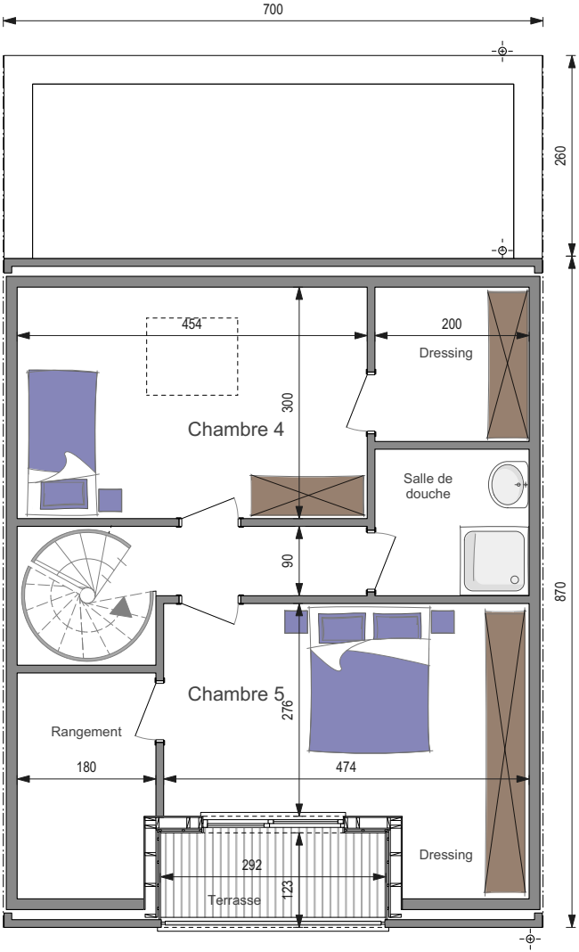
2 ème ÉTAGE
