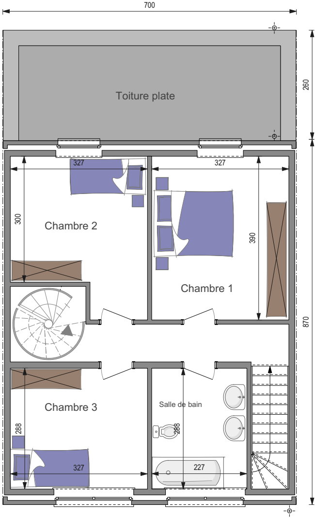
1 er ÉTAGE
